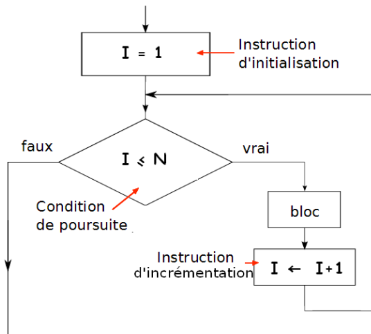
Organigramme de la boucle "Pour I variant de 1 à N par pas de 1 faire ... "
